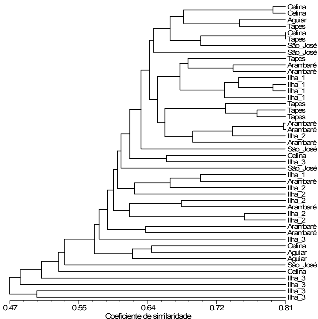
Figura 3 – Agrupamento dos 46 indivíduos das oito populações de butiazeiros através da matriz de similaridade calculada pelo coeficiente de Jaccard utilizando o método UPGMA com base em 199 marcadores AFLP. O coeficiente de correlação cofenético ( r ) é = 0,83. Pelotas, 2008.
